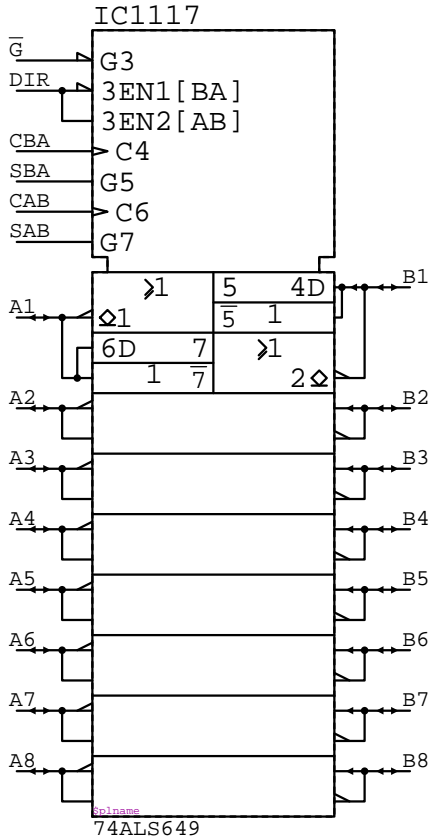
74ALS649
