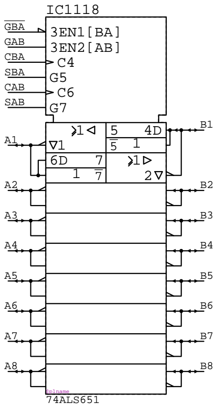
74ALS651
