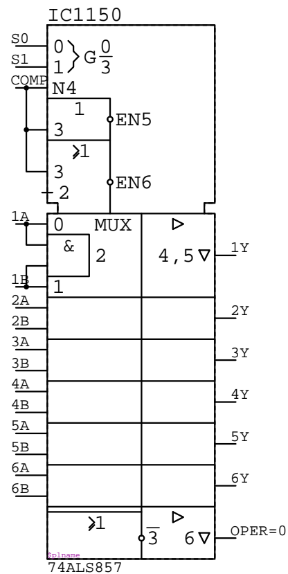
74ALS857
