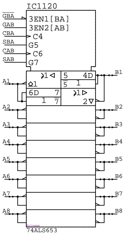
74ALS653
