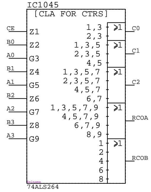
74ALS264
