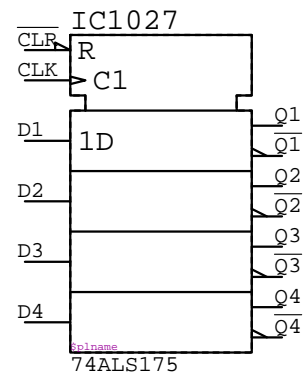
74ALS175
