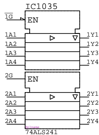
74ALS241
