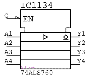
74ALS760
