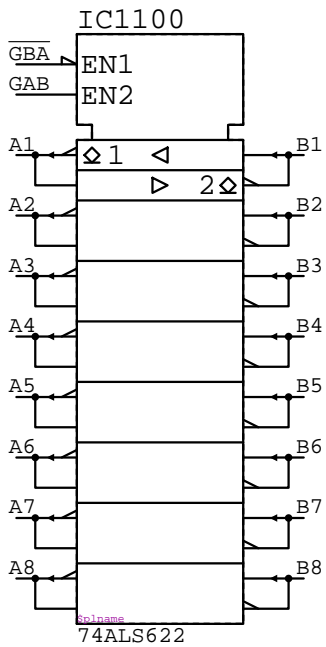
74ALS622
