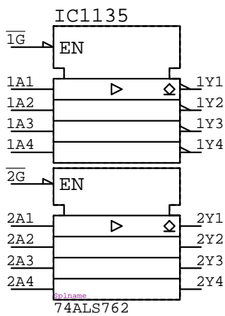
74ALS762
