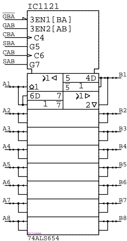
74ALS654
