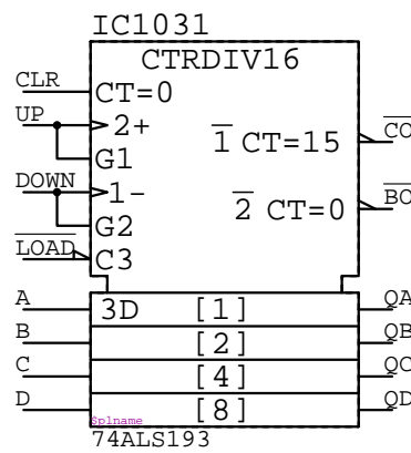
74ALS193
