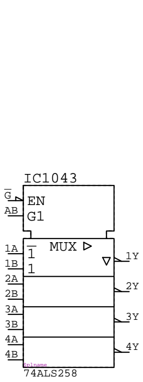
74ALS258
