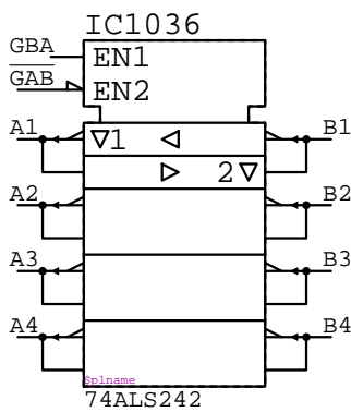
74ALS242
