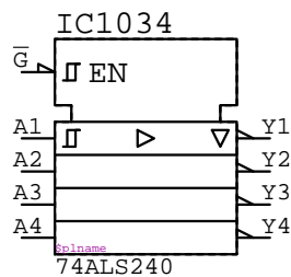
74ALS240
