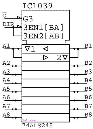
74ALS245
