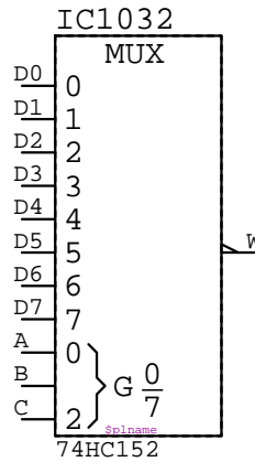
74HC152
