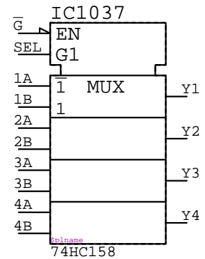
74HC158
