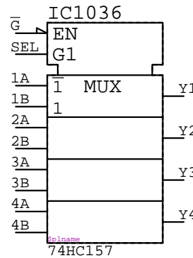
74HC157
