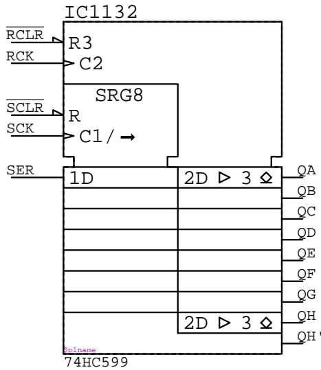
74HC599 IC?????
