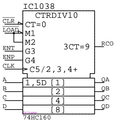
74HC160
