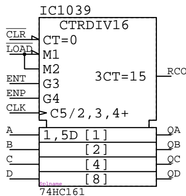
74HC161
