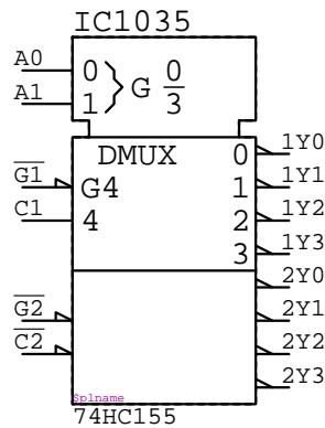
74HC155
