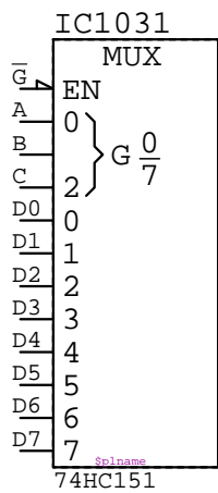
74HC151
